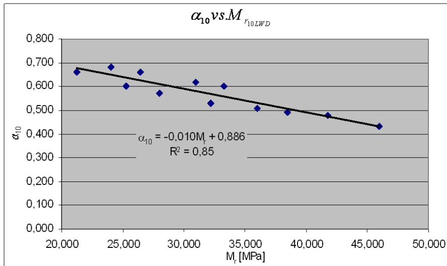
Figura 8. Gráfica coeficiente vs. M_r para masa de 10 kg
