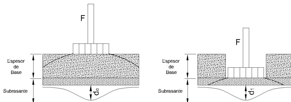
Figura 3. Forma de medición propuesta (Fuente: Elaboración propia)
