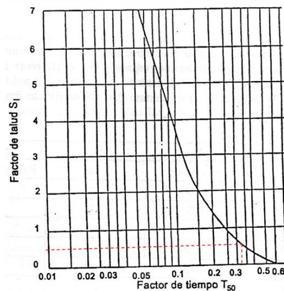
Figura 6. Factor de tiempo de drenaje del 50 % (Fuente: EICAM, 1998)
