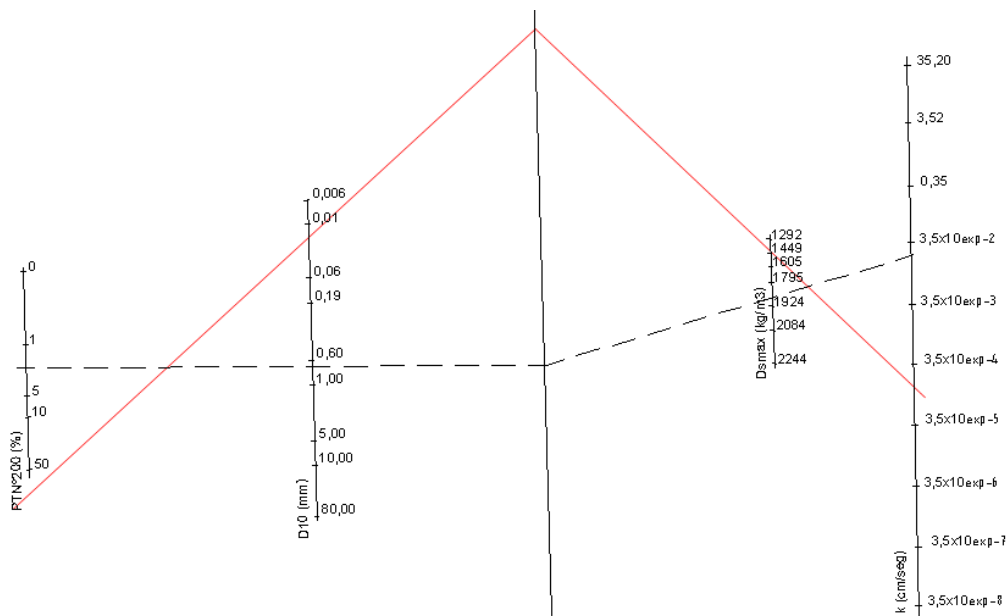
Figura 5. Abaco para estimar permeabilidad (Fuente: EICAM, 1998)
